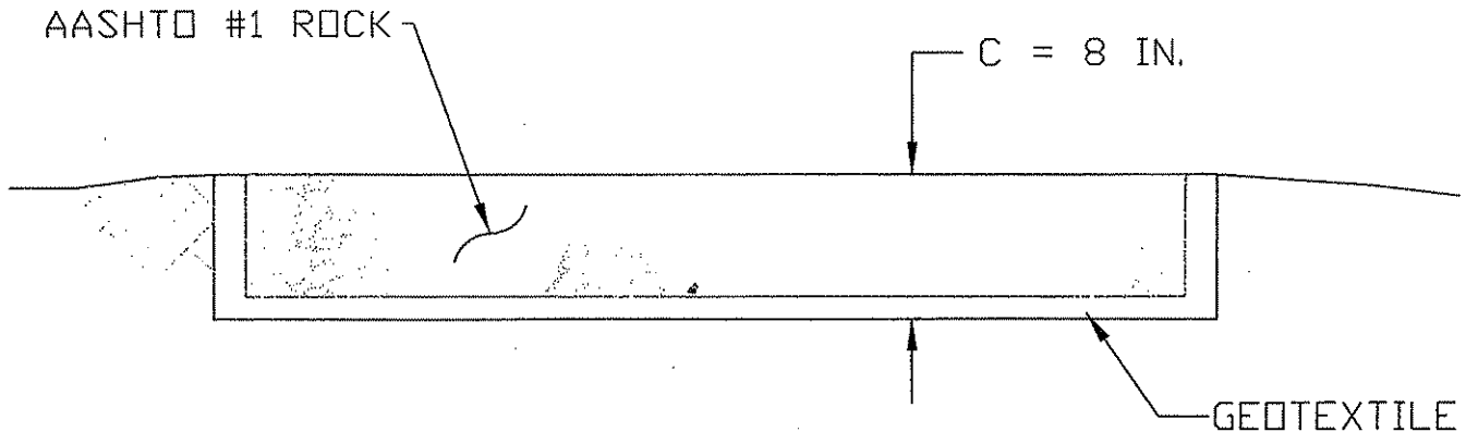
SECTION A-A
